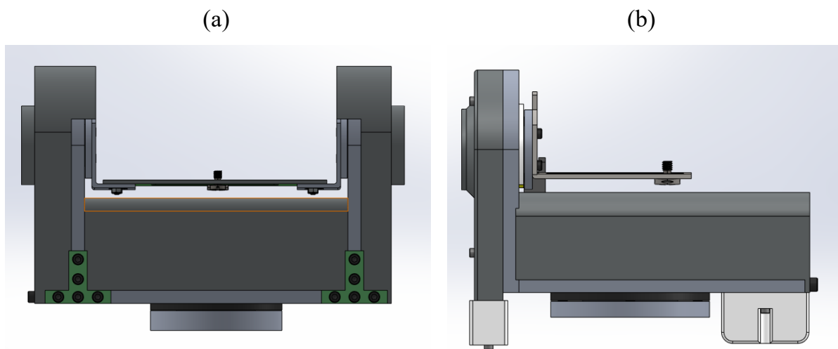
Hình 3.3: (a) Kết cấu robot hình chữ U, (b) kết cấu robot hình chữ L
